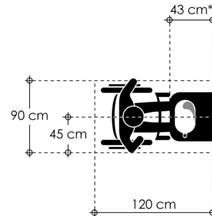
Figura No.4 Espacio mínimo para uso de bebedero por persona con silla de ruedas
