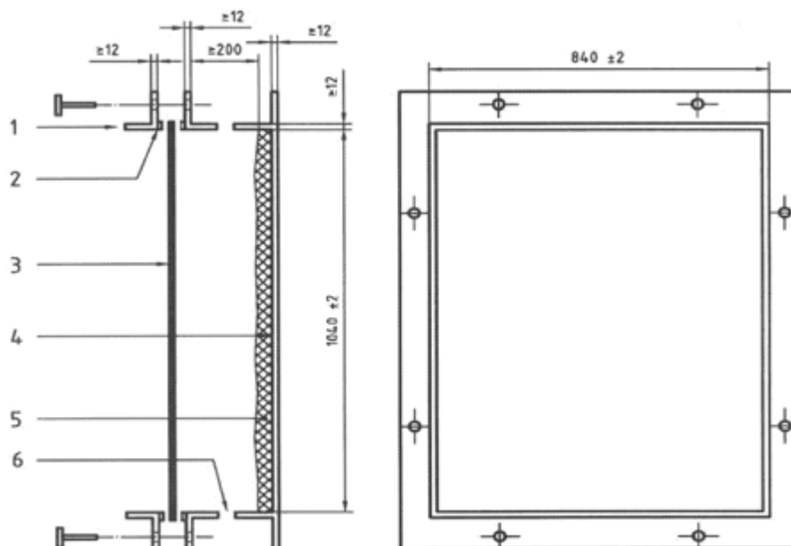
VISTA SUPERIOR DEL BASTIDOR
