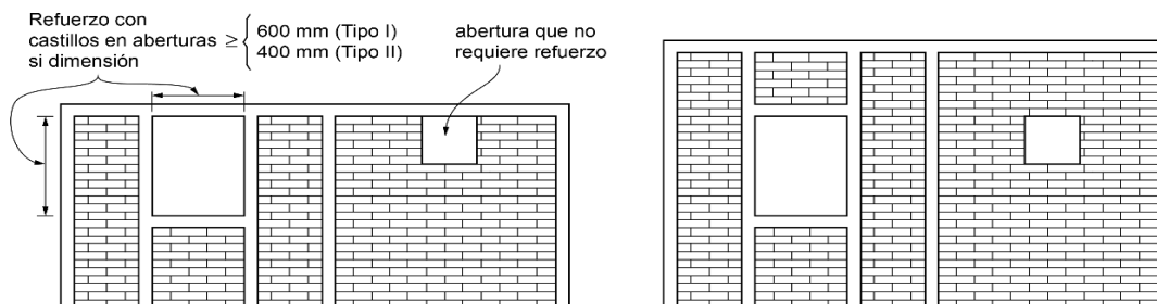
Figura 5.1.3 Refuerzo en el perímetro de aberturas
