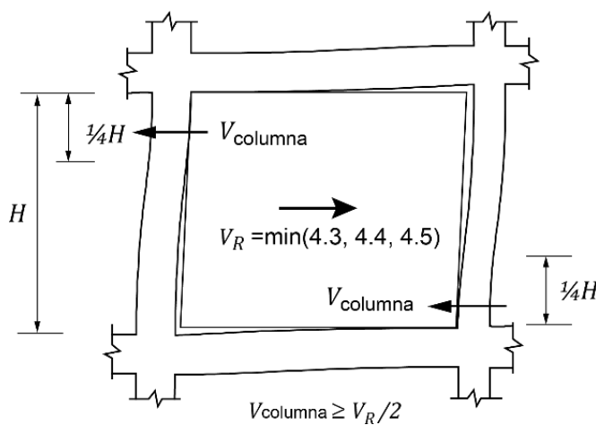
Figura 4.8.1 Interacción marco–muro diafragma
