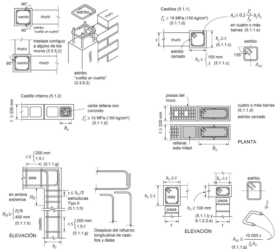
Figura 5.1.2 Castillos y dalas
