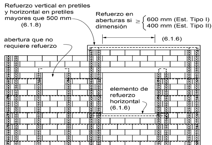
Figura 6.1.3 Refuerzo en aberturas y pretilas
