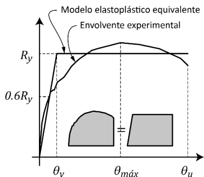
Figura A.8.2 Modelo elastoplástico equivalente
