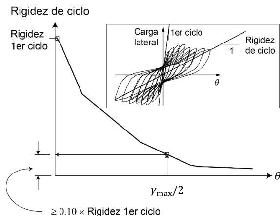
Figura A.8.1 Degradación de rigidez de ciclo
